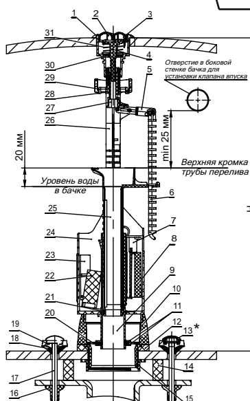
Рис. 2 - Клапан выпуска
